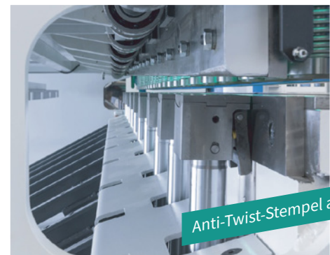
Anti-Twist-Stempel abgesenkt
